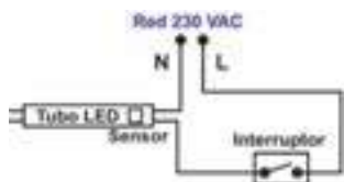
Esquema Conexión Tubo LED con Sensor-Radar:
