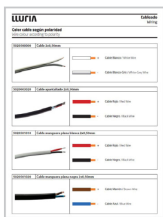
Polaridad cables
