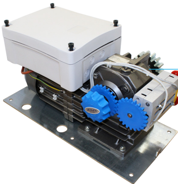
RÉDUCTEUR ET STRUCTURE CAPABLE DE SUPPORTER DE GRANDS EFFORTS. REDUCTOR Y ESTRUCTURA MECÁNICA CAPAZ DE SOPORTAR GRANDES ESFUERZOS.
